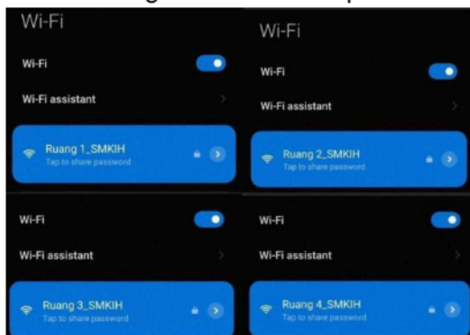
Gambar 21 SSID
