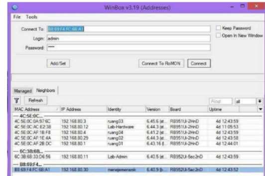
Gambar 4 Halaman Login
