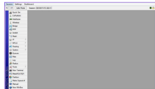
Gambar 5 Dashboard Utama
