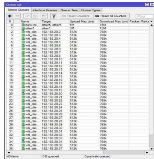
Gambar 18 QoS
